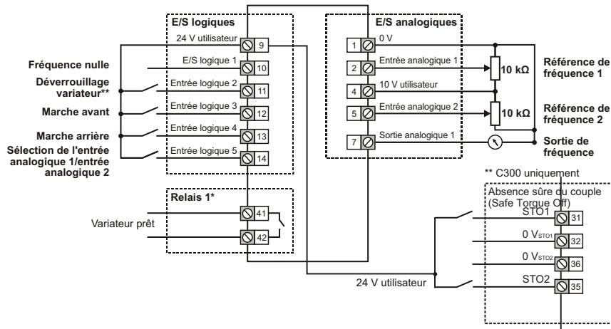
Figure 1-12 Connexions de contrôle
