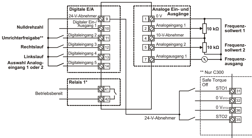
Abbildung 1-13 Steueranschlüsse
